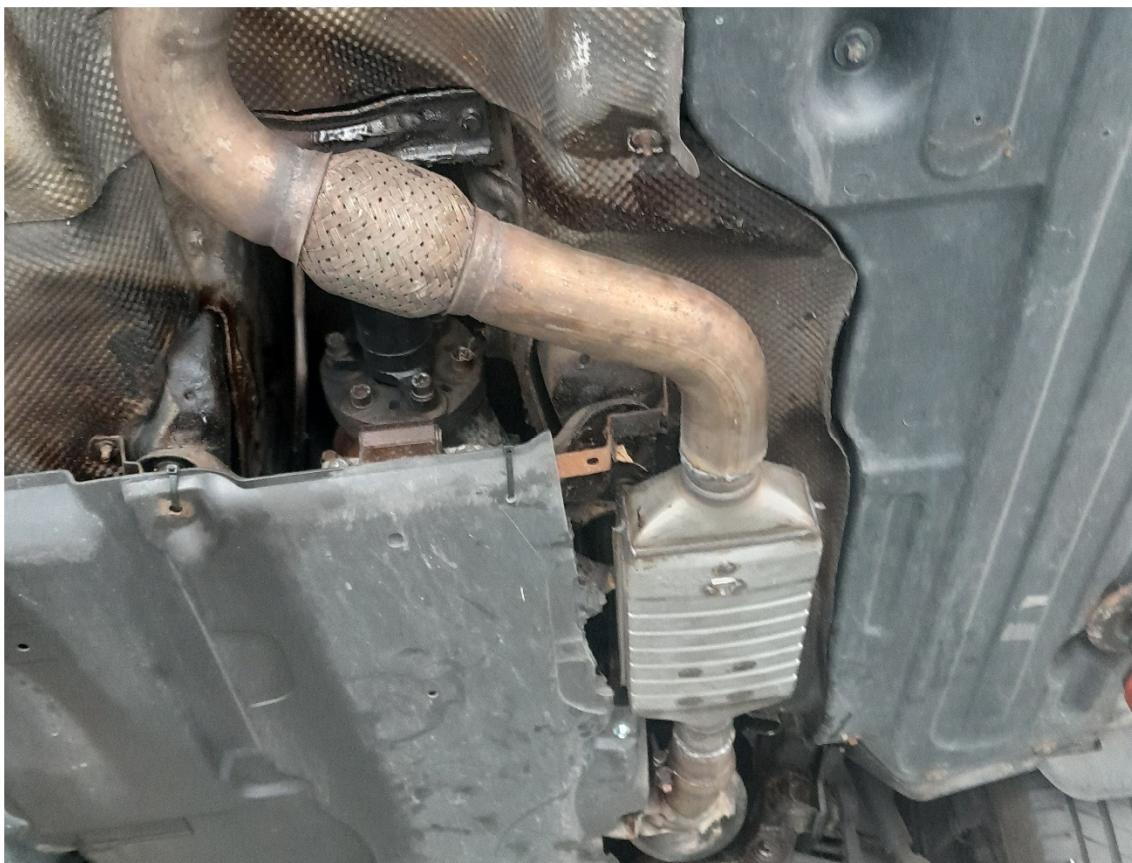
Eksempel 3) Montering på højre side af gearkasse, lige efter katalysator. Her MB E320 3,0 EURO 4. Det kræver modificering af beslag til ophæng på gearkasse, afkortning af forrør efter flexrør, samt modificering af bundplade.
